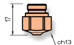
Kupfer-Düse
