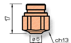
Kupfer-Düse
